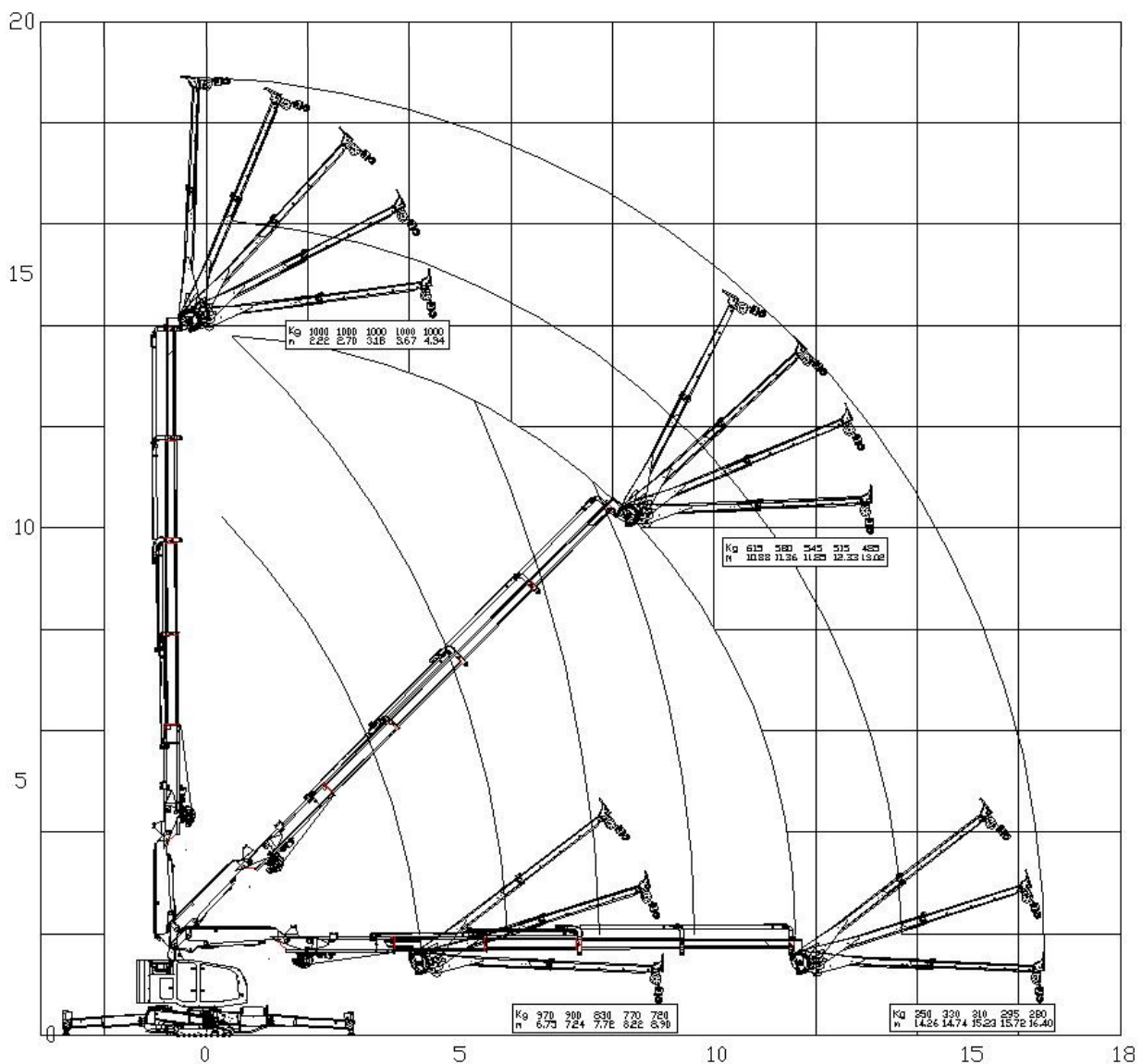
Hijslast tabel met jib volledig gestempeld
